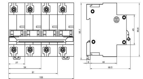
Рисунок 3. Габаритные, установочные, присоединительные размеры выключателей
