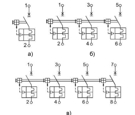
Рисунок 4. Принципиальные электрические схемы выключателей
