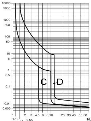
Рисунок 5. Защитная характеристика в цепи переменного тока по ГОСТ Р 50345
